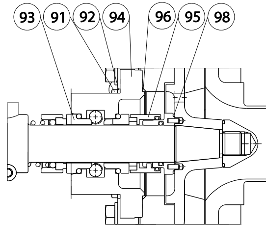
Figuur 6 Mechanische asafdichting Q12.
